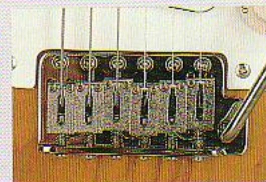
トレモロには、サスティーンの良さが特徴のスティールサドルを採用
