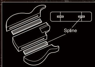
スプラインジョイント構造3ピースボディ
