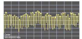
実際のスペクトラムスキャン結果。従来16チャンネルの運用であった周波数帯域で47チャンネルを運用できていることがわかります。(米国の周波数運用例)
